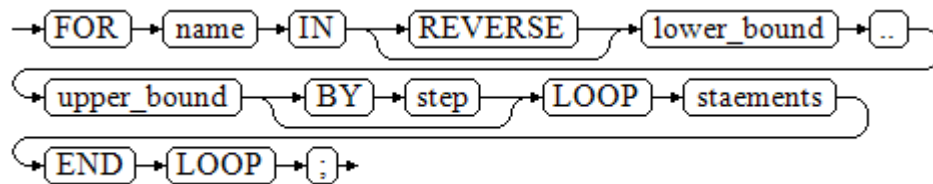
图 12-22 for_loop::=
