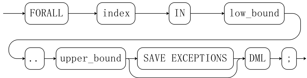
图 12-24 forall::=
