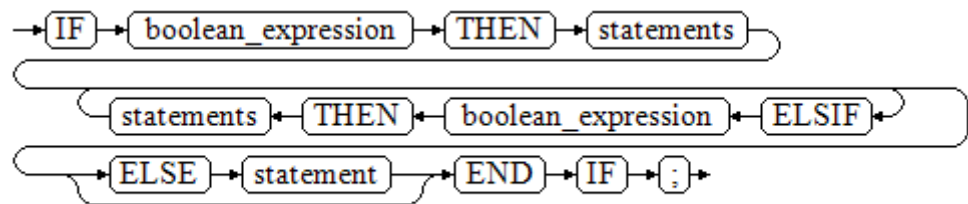
图 12-19 IF_THEN_ELSEIF_ELSE::=
